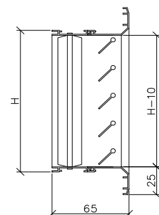
РВ 2565-2М
