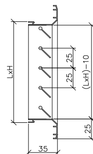
РВ 2535-1Ж
