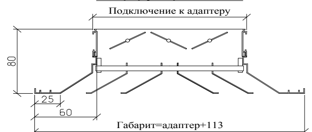
Диффузор ПДК+R
