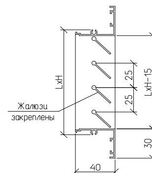
РВ 3040-1Ж
