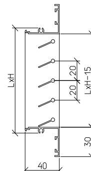
РВ 3040-1
