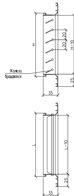
РВ 2535-1
