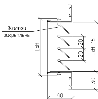
РВ 3040-1П
