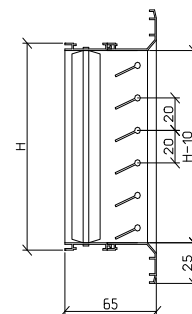
РВ 2565-2
