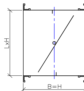
Дроссель-клапан ДК
