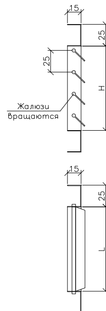
РВ 1525-1
