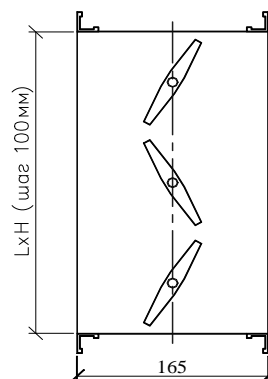
ВРК
