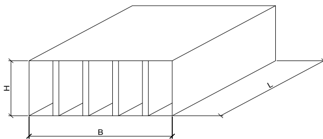
Шумоглушитель ШПК
