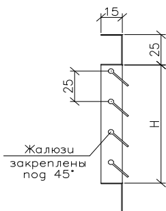
РВ 1525-1Ж
