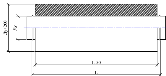
Шумоглушитель ШПК
