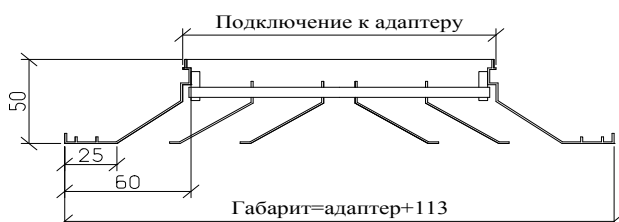
Диффузор ПДК
